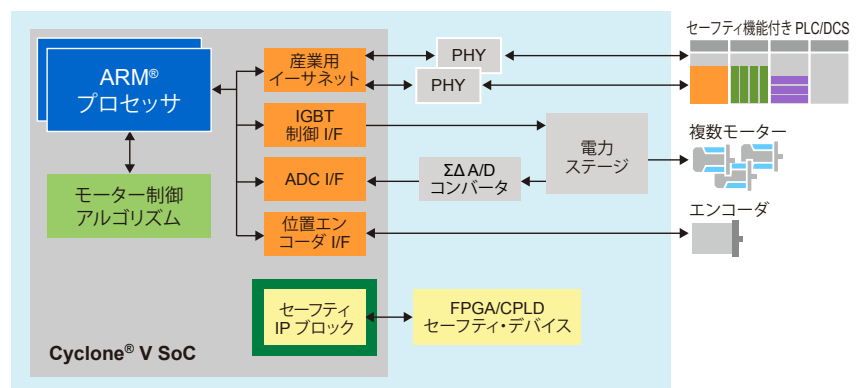
図1、「ワンチップ・ドライブ装置」: Cyclone V SoC FPGA は、ARM プロセッサを含みます。その他、モーター制御アルゴリズム、I/O ロジック、産業用イーサネット・プロトコル、およびセーフティ・エレメントも統合可能です。
