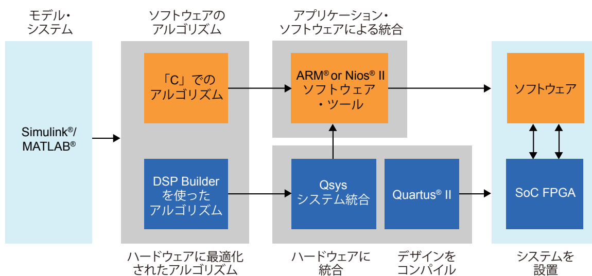
図 2：SoC FPGA ドライブ装置システム向けにシステム・レベルで最適化されたデザイン・フロー
