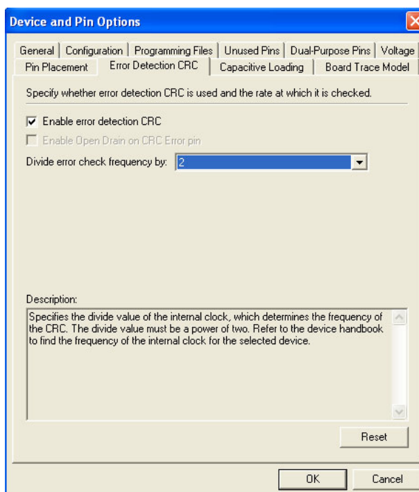
図 11-3. Quartus II ソフトウェアにおけるエラー検出 CRC 機能のイネーブル
