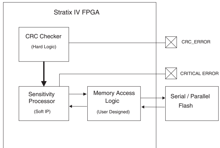
図 11-1. 重大エラー検出実装のブロック図
