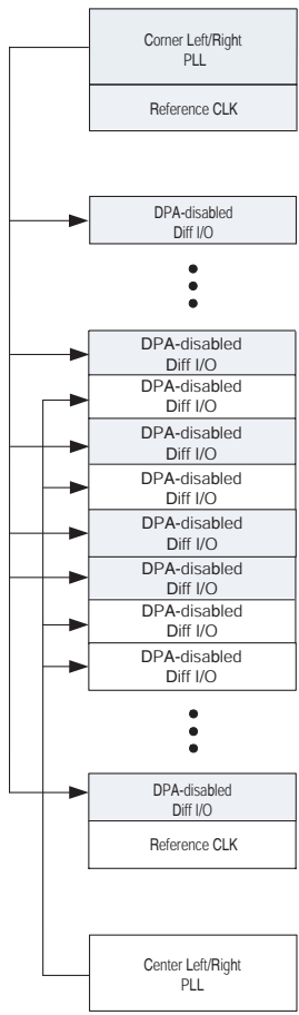
図 8-21. コーナーおよびセンター・レフトおよびライト PLL でドライブされるチャンネルのインタリーブによる DPA がディセーブルされた差 I/O の無効な配置
