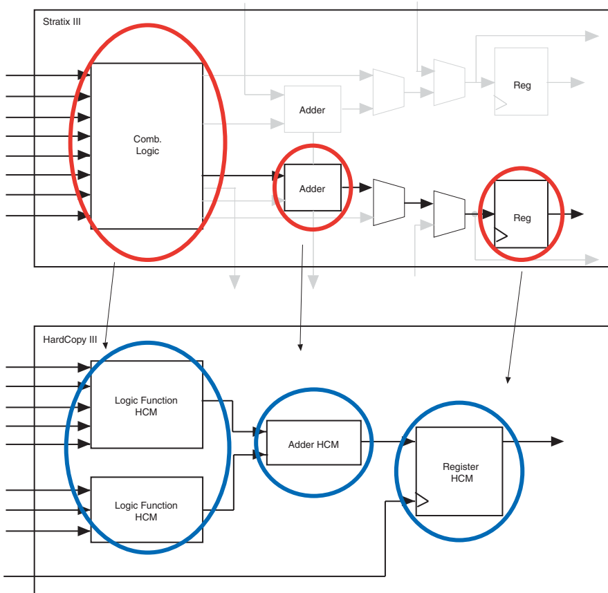
図 2-2. HCell マクロにマップされた ALM ファンクション例
