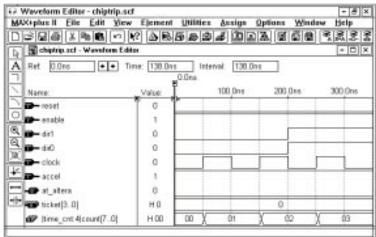
図3 MAX+PLUS II の波形エディタ
